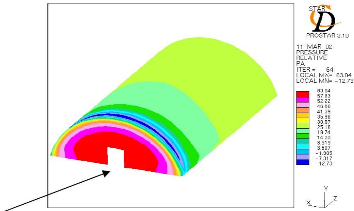
Рисунок 1 – Поле давлений на поверхности ангара
