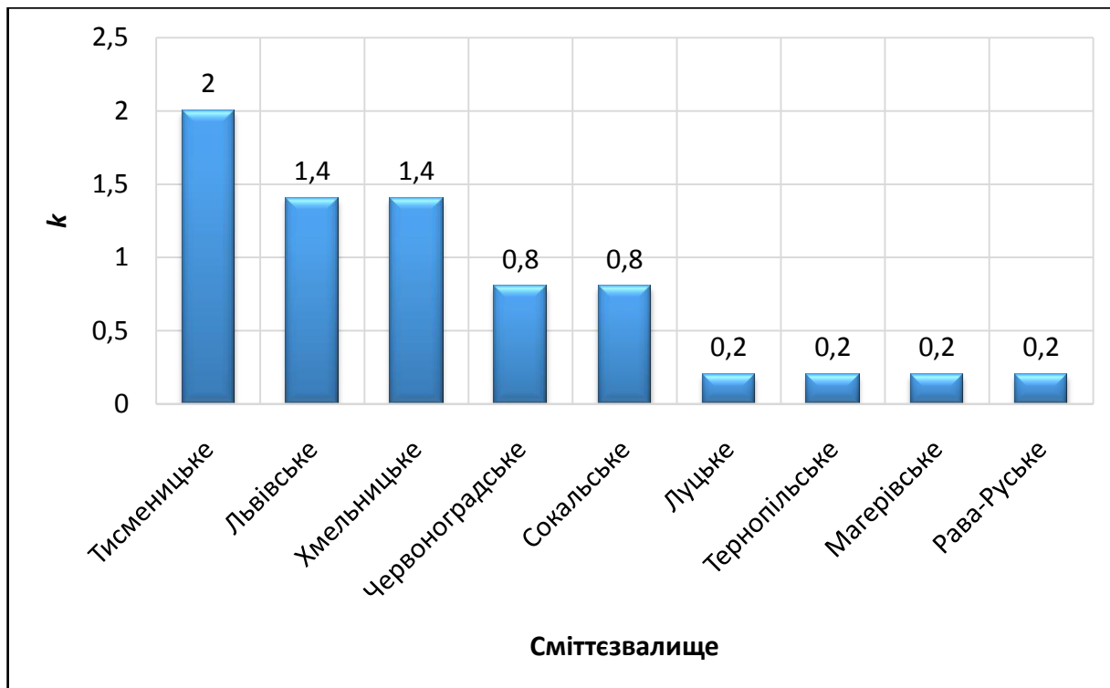
Рис. 2. Коефіцієнти безпеки досліджуваних сміттєзвалищ з урахуванням поведження із фільтратом
