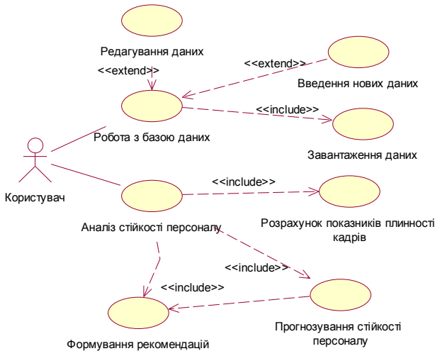
Рис.1. Діаграма варіантів використання модуля Список використаних джерел:
