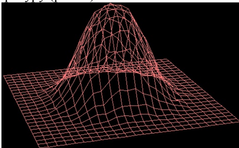
Рис. 3 Тривимірний графік температури при об'ємі комірок 20 на 20
