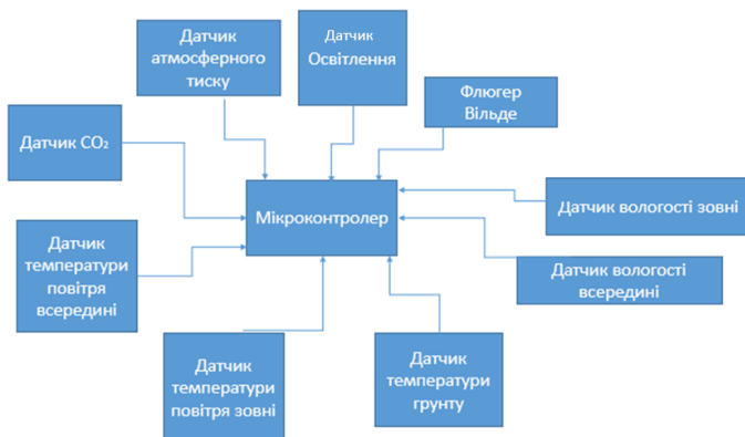
Рис. 1 – Структурна схема автоматизації теплиці з алгоритмом прогнозування
